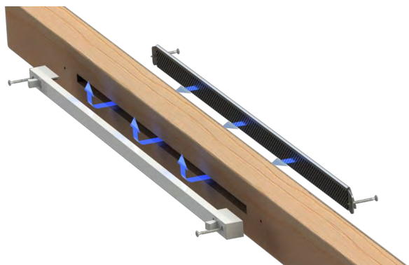
Spalteventil Vannese
